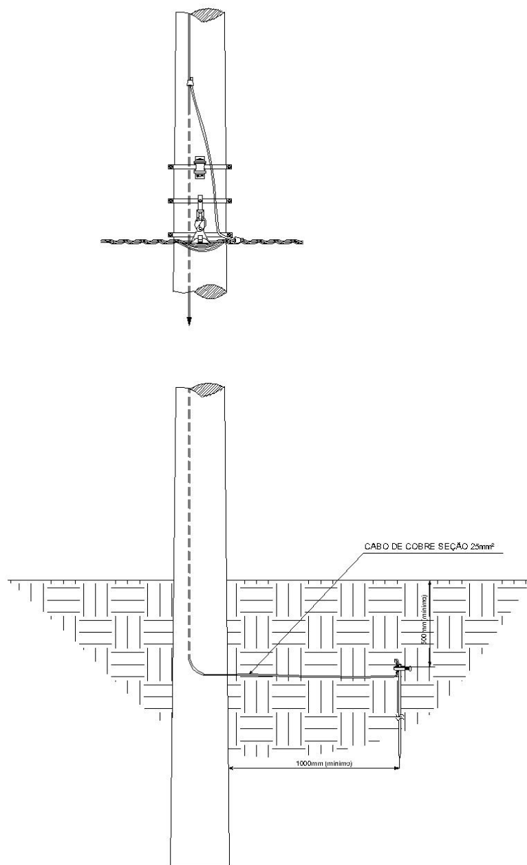
Figura 21 - Aterramento - Neutro
