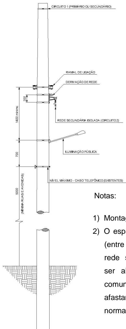
Figura 1 – Instalação básica
