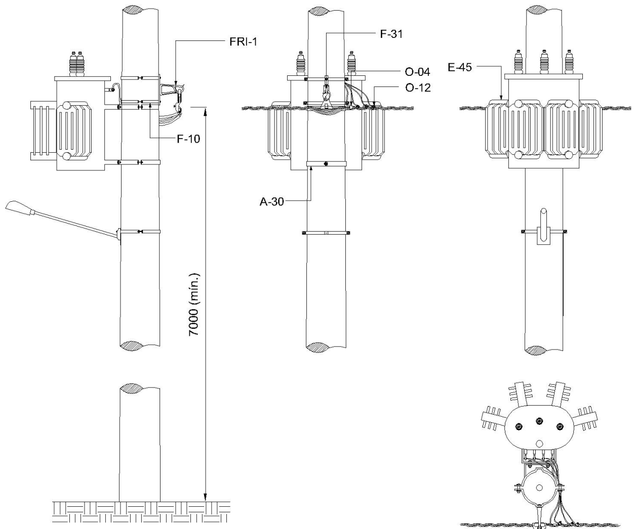
Figura 13 - Instalação de transformador SITR
