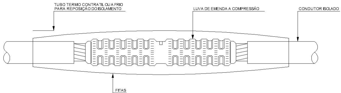
Figura 23 - Emenda reta do cabo - Maneira 2
