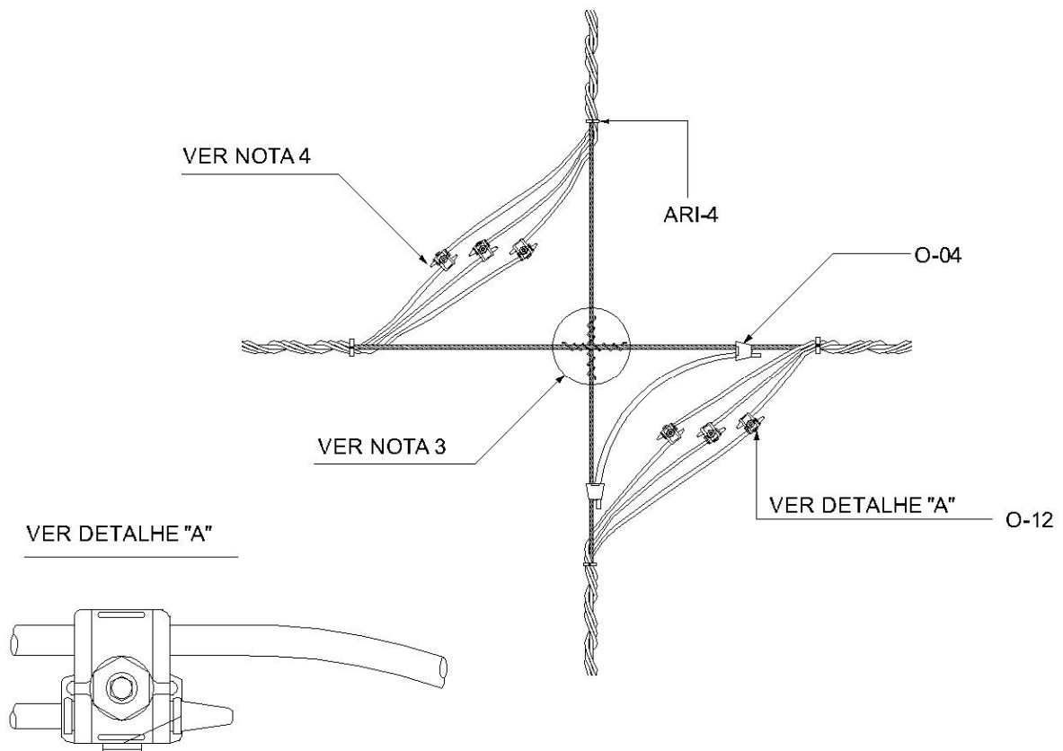
Figura 11 - Estrutura cruzamento sem conexão no vão
